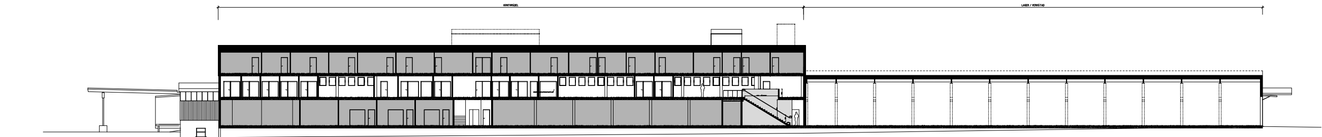
PRINCIPSEKTION B-B NYTT
